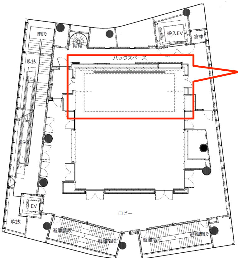
【ステージ平面図】
